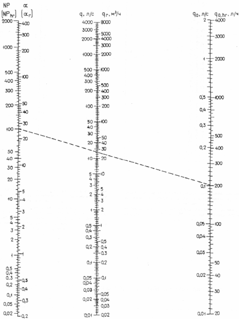
Черт. 4. Номограмма для определения секундных и часовых расходов воды в зависимости от NP ( NP_{hr} ) при различных значениях q_0 , л/с, и q_{0,hr} , л³/ч
